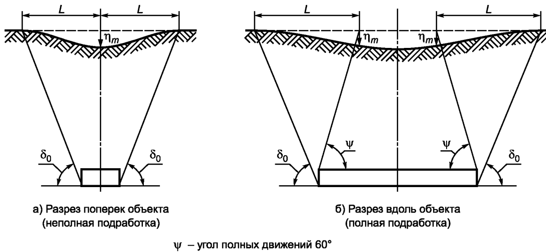
Рисунок Р.1 — Основные параметры мурды сдвига
